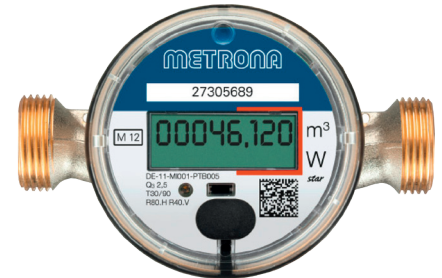
Contador de agua vía radio Metrona star
